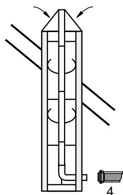
C93x sistema estanco Sistema DN80/185 horizontal y DN80 vertical
