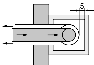
C33x sistema estanco en el patinillo de obra DN80/125
