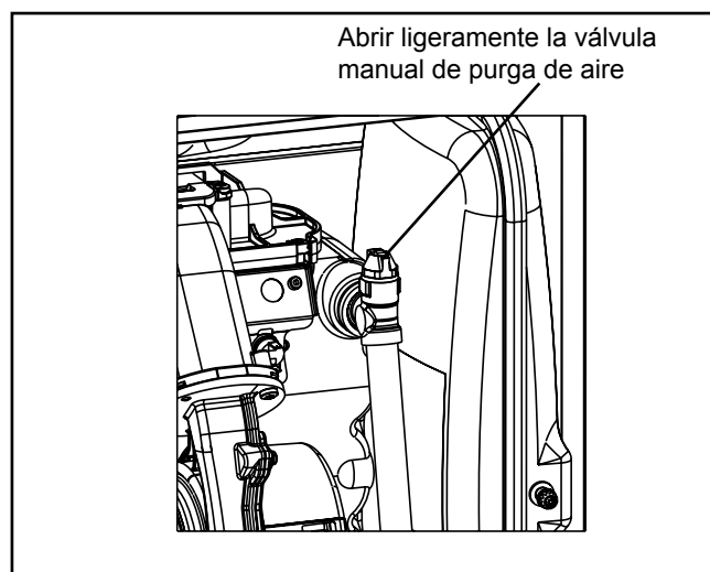
Figura: Válvula manual de purga
