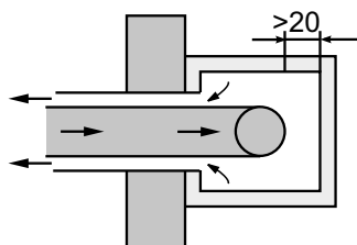
C93x sistema estanco en patinillo de obra DN80
