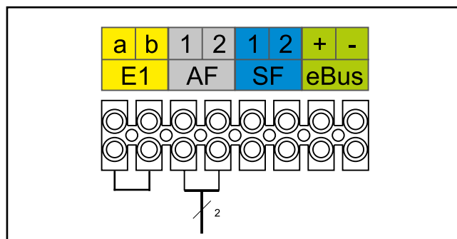
Figura: Conexión de sonda de temperatura exterior
