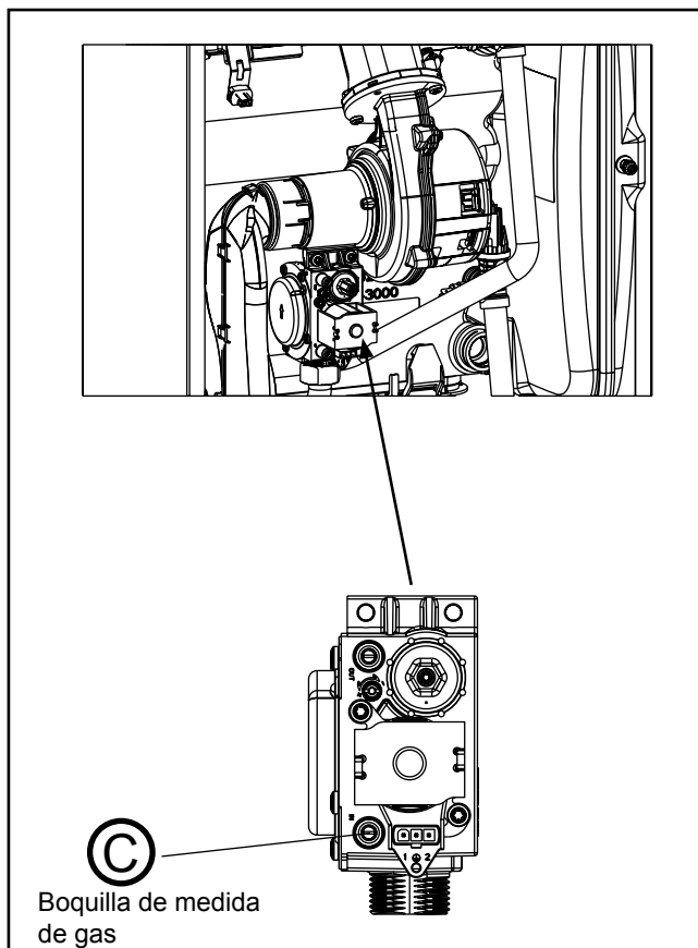
Figura: Comprobación de la presión de conexión de gas
