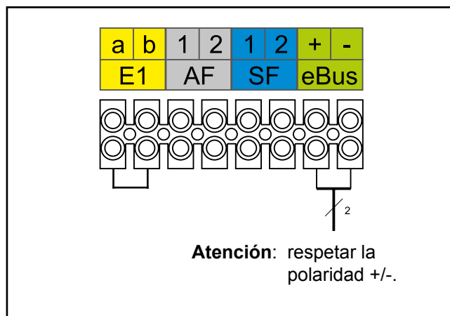
Figura: Conexión de accesorio de regulación digital de Wolf (interfaz de eBus)
