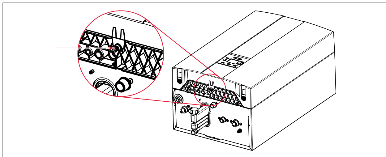
Fig. 1.1 Abrir el revestimiento
