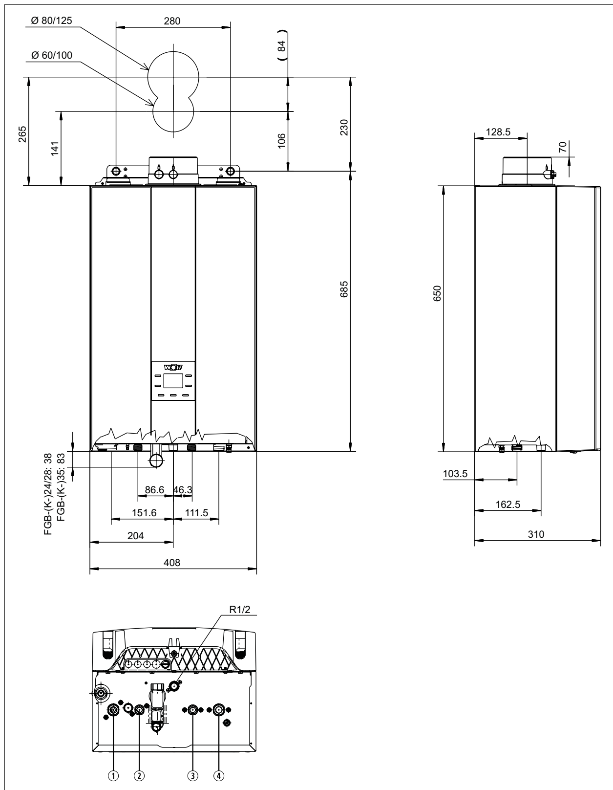
Fig. 1.1 Dimensiones FGB-(K-)
