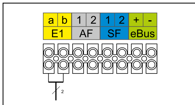
Figura: Conexión entrada E1
