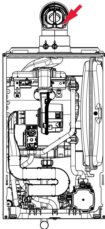
Fig. 1.1 Llenar el sifón a través del tubo de gases de combustión
