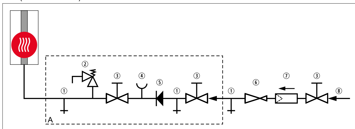
Fig. 1.2 Conexión de agua fría según DIN 1988
