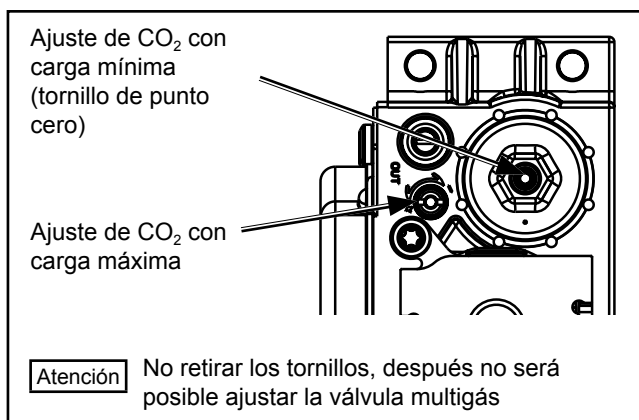
Figura: Válvula multigás
