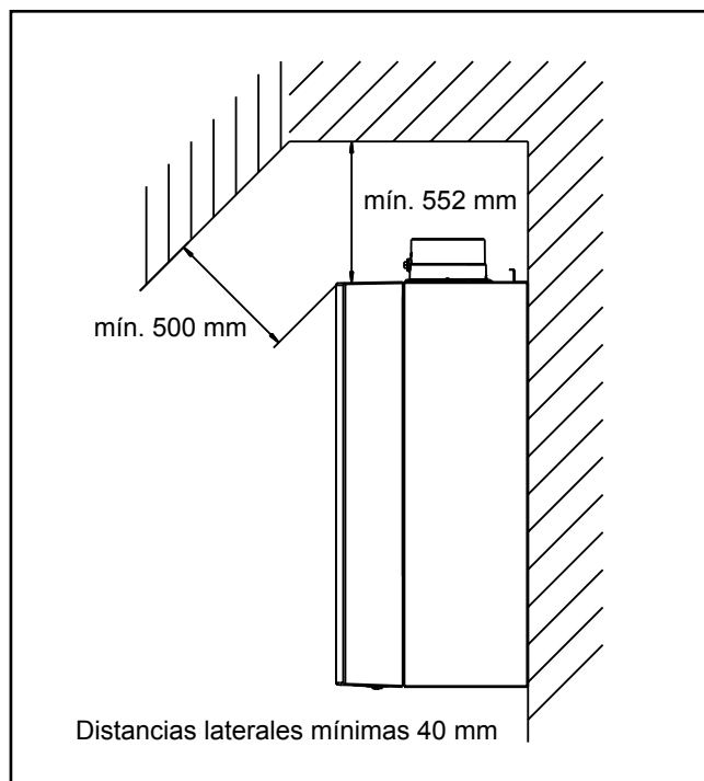
Figura: Distancias mínimas
